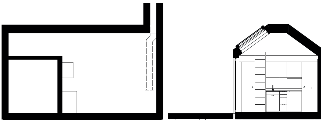
Ateljé 25 KOMPLETT Alt. 1 - Sektioner
