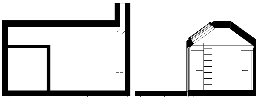
Planlösning INDIVIDUELL - Sektioner
