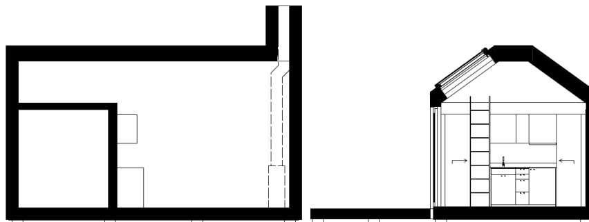
Planlösning KOMPLETT Alt. 1 - Sektioner
