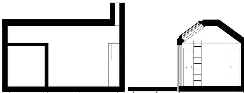
Ateljé 25 KOMPLETT Alt. 2 - Sektioner
